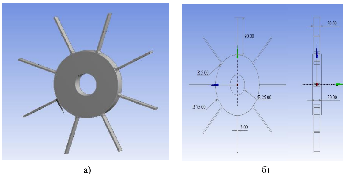
Рисунок 1 – Трехмерная модель и размеры рабочего колеса паровой турбины: а – трехмерная модель колеса; б – размеры колеса, мм
