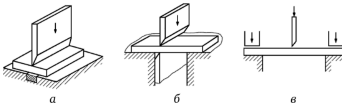
Рисунок 4 – Актуальные виды процесса резания: а – давлением относительно прочной основы; б – контрножами; в – свободное.
