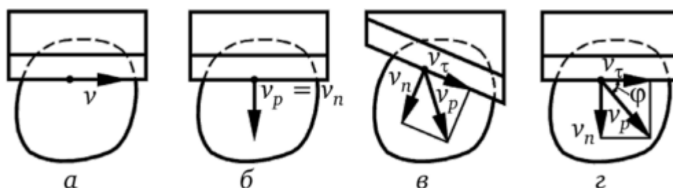
Рисунок 5. Схема перемещения ножа относительно обрабатываемого продукта: а – касательное перемещение; б – нормальное перемещение; в – наклонное перемещение; г – перемещение под углом к режущей кромке.
