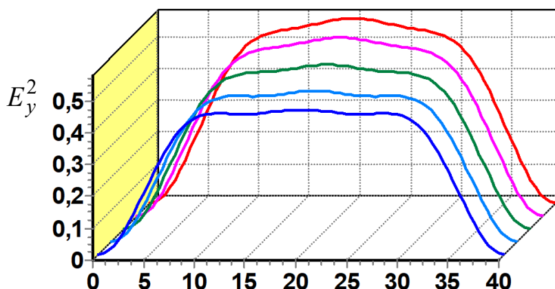
Рисунок 2 – Распределение электрической компоненты TE_{10} - волны в сечении материала
