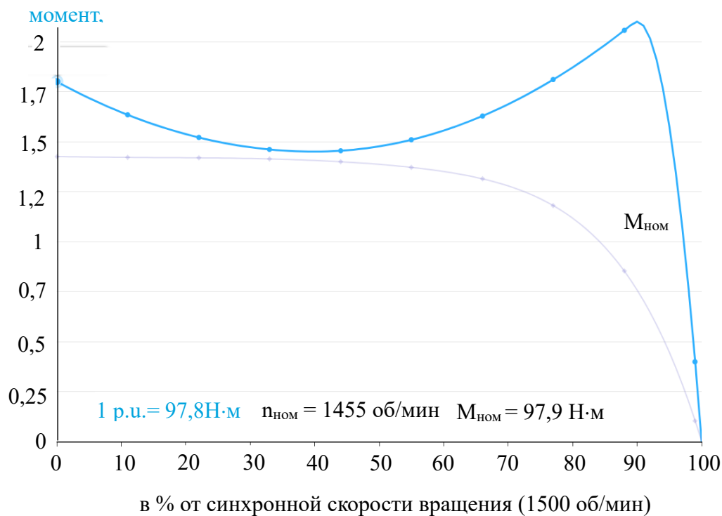
Рисунок 4 – Механическая характеристика инверторного индукционного двигателя (IE1) фирмы WEG: P_{\text{ном}} = 15 кВт, U_{\text{ном}} = 380 В и f_{\text{сети}} = 50
