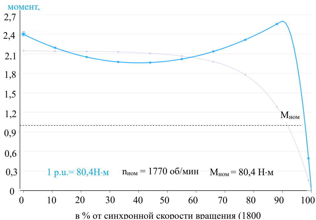
Рисунок 3 – Механическая характеристика инверторного индукционного двигателя фирмы WEG: P_{\text{ном}} = 15 кВт, U_{\text{ном}} = 230/460 В и f_{\text{сети}} = 60 Гц
