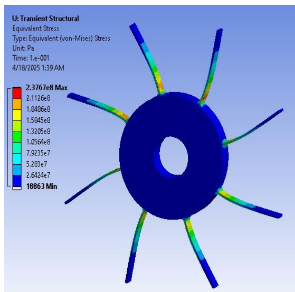
Рисунок 4 – Результаты расчета НДС рабочего колеса: а – без трещины; б – с трещиной (10%); в – с трещиной (20%); г – с трещиной (30%)
