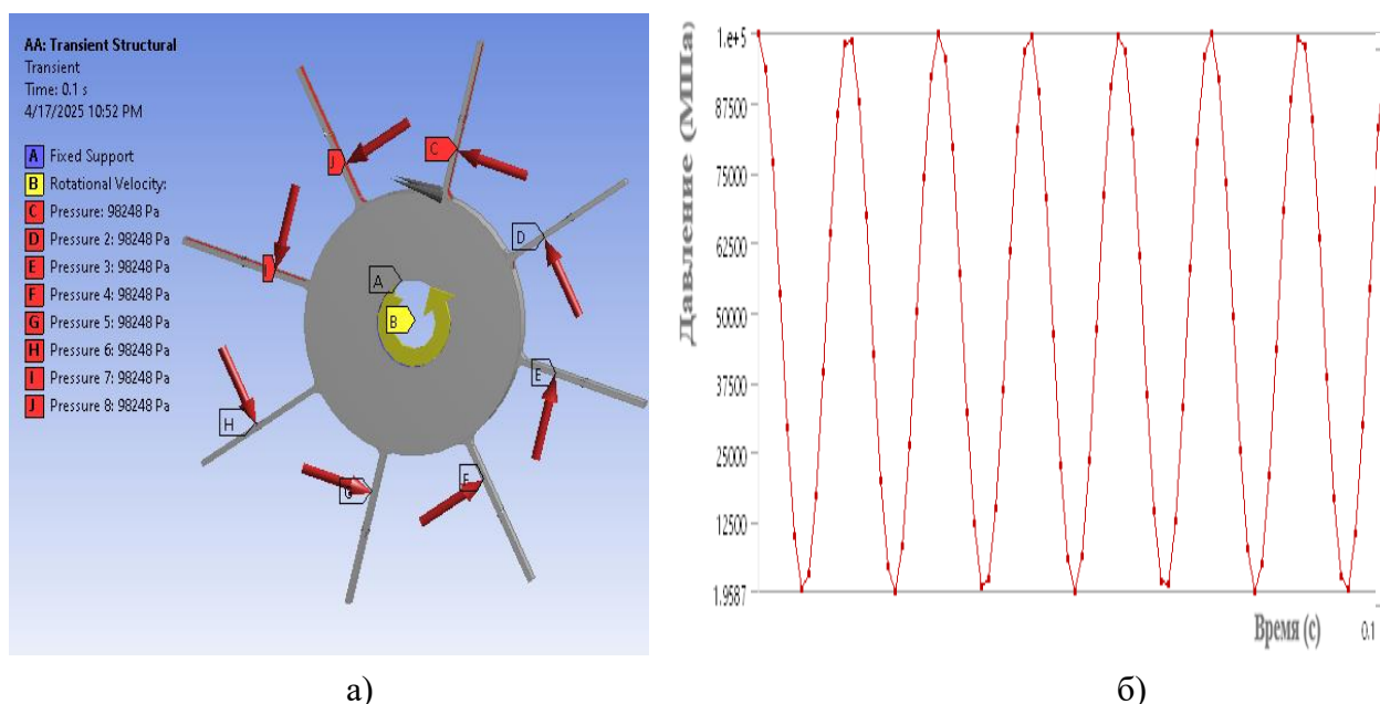
Рисунок 2 – Граничные условия задачи: а – схема нагружения рабочего колеса; б – динамическое давление, приложенное к поверхности лопаток
