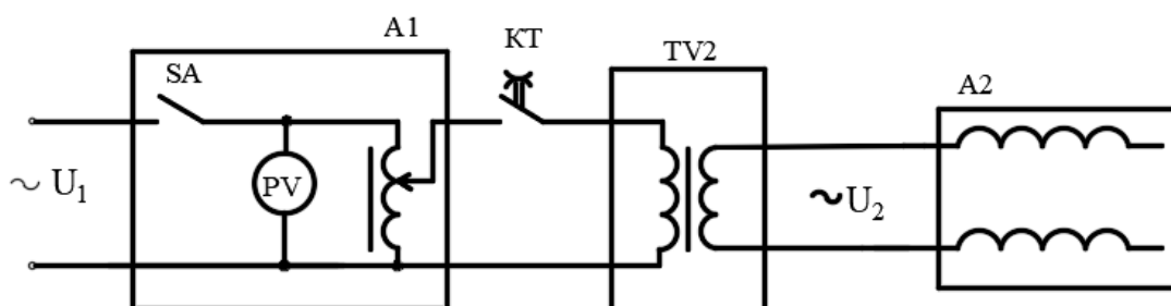
Рисунок 1 – Структурная схема экспериментальной установки: U_1 – переменное сетевое напряжение; SA – переключатель; PV – вольтметр; A1 – ЛАТР (лабораторный автотрансформатор регулируемый); KT – реле времени; TV2 – повышающий трансформатор; A2 – секция электродов
