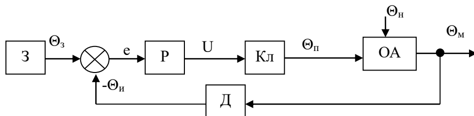
Рисунок 3 – Функциональная схема контура регулирования температуры пастеризации молока: \mathcal{Z} – задатчик, Р – регулятор (контроллер), Кл – клапан, ОА – объект автоматизации, Д – датчик
